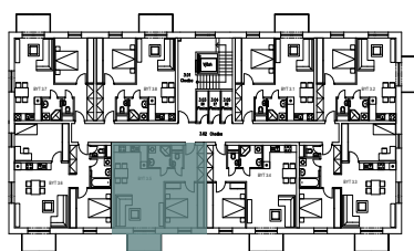
PÔDORYS PODLAŽIA
