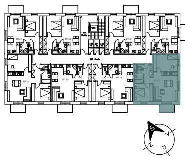
PÔDORYS PODLAŽIA
